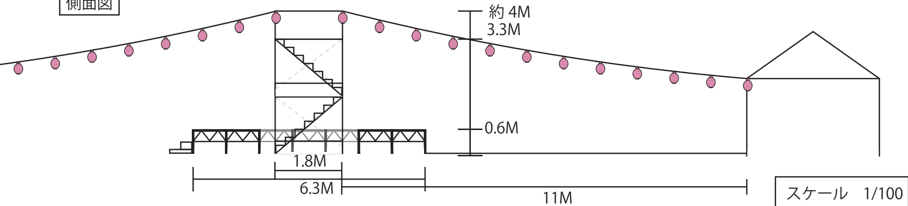
側面図
