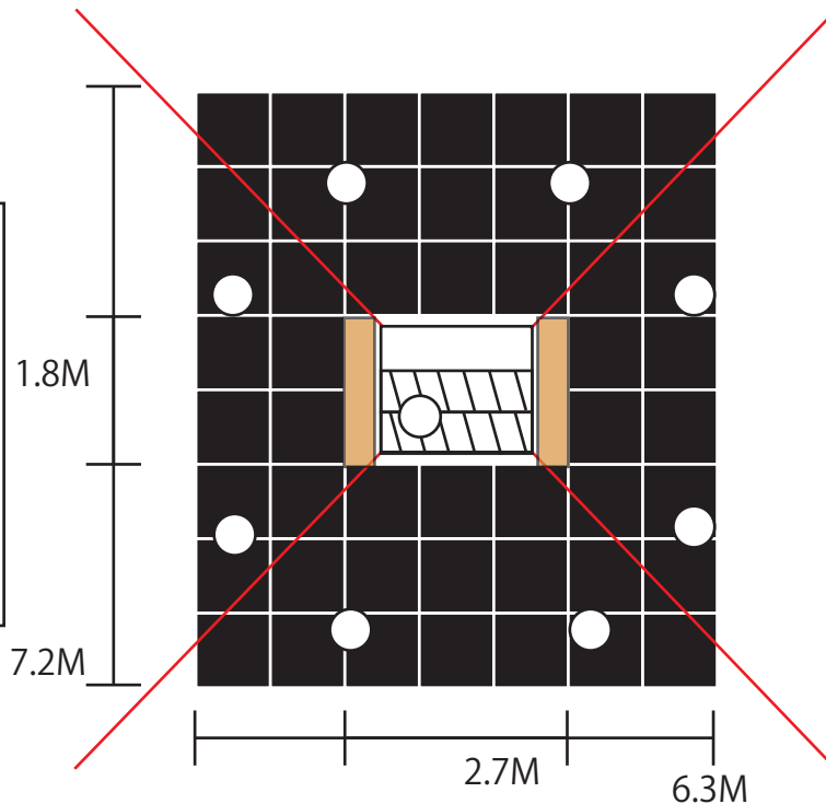
ステージ上面図
